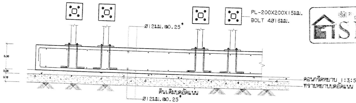
ขยายฐานราก 1:20
