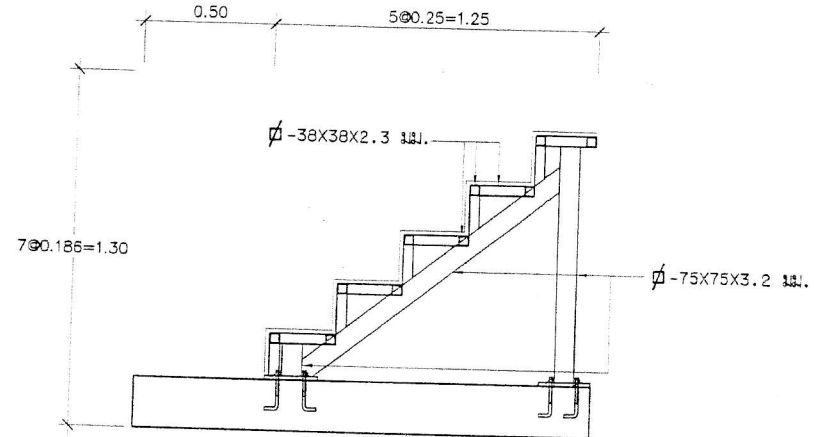
ขยายบันได 1:20
