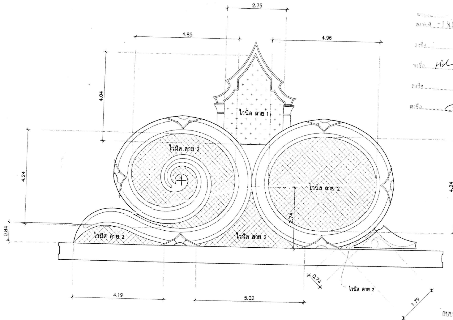
แบบขยายขนาดวาณิช มาตราส่วน 1 : 75
