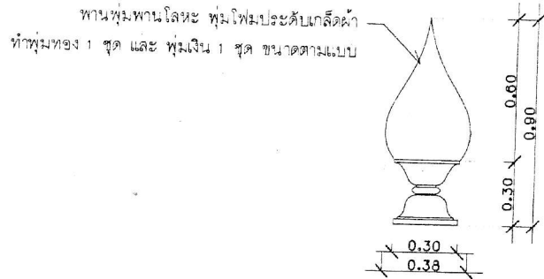
แบบขยายพานพุ่มทอง-พุ่มเงิน มาตราส่วน 1:20
