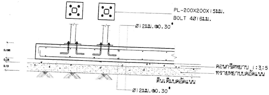
ขยายฐานรากบันได 1:20
