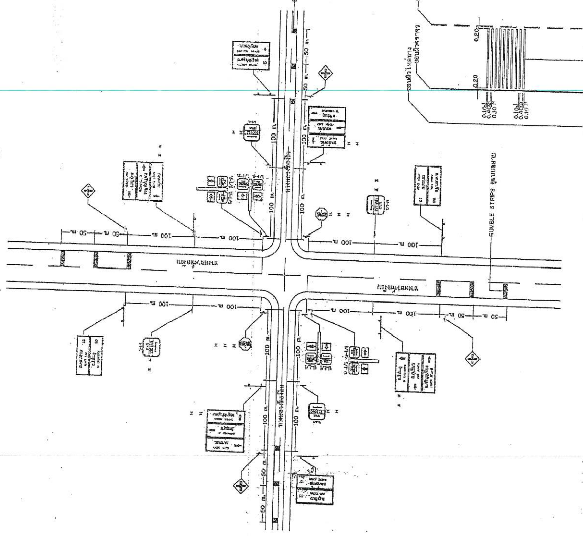
แผนผังการติดตั้งป้ายจราจรบริเวณสี่แยก ( เชื่อมทางหลวงท้องถิ่น )
