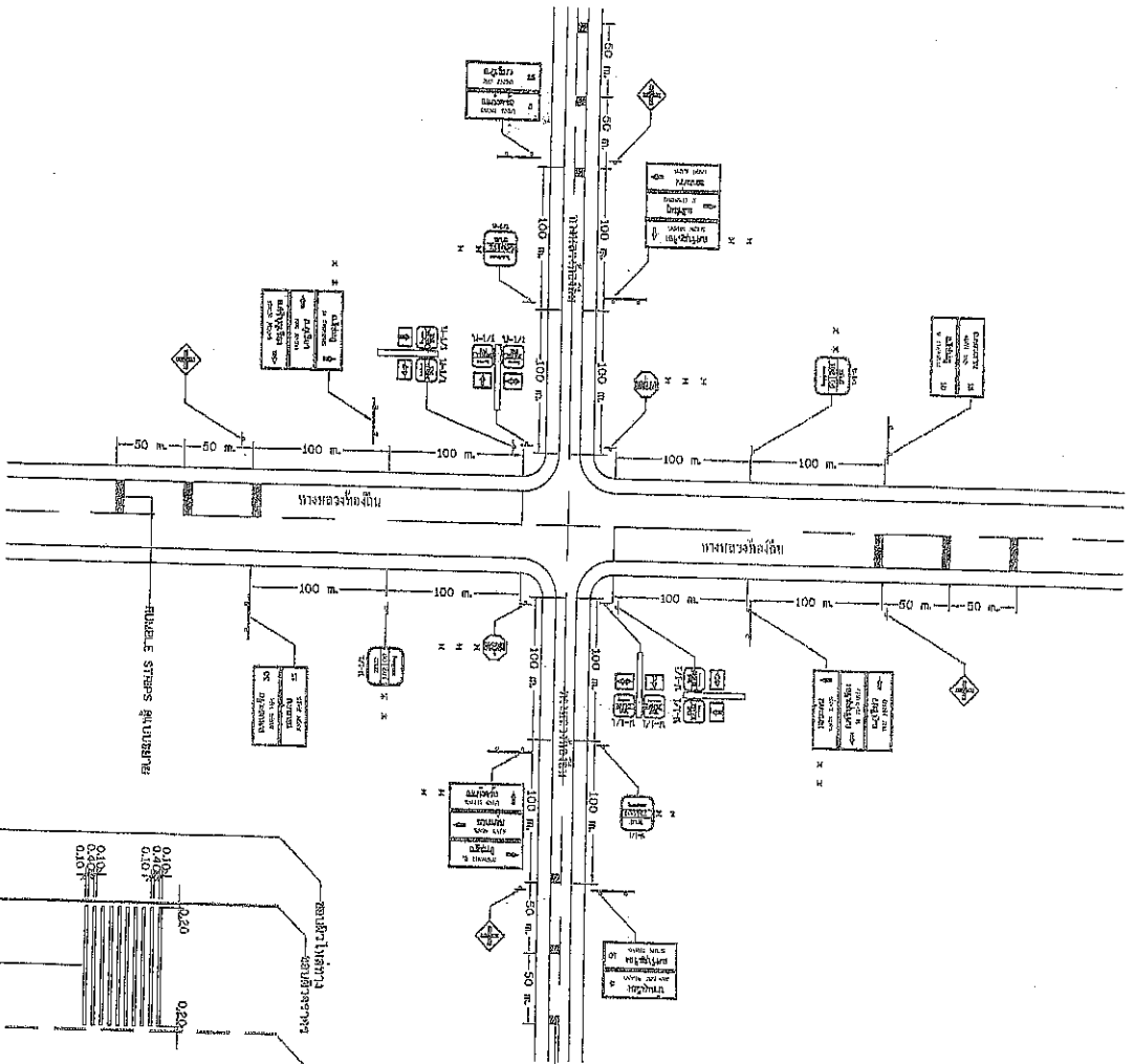
แผนผังการติดตั้งป้ายจราจรควบคุมสัญญาณจราจร ( ใช้ตามทางหลวงชนบท )
