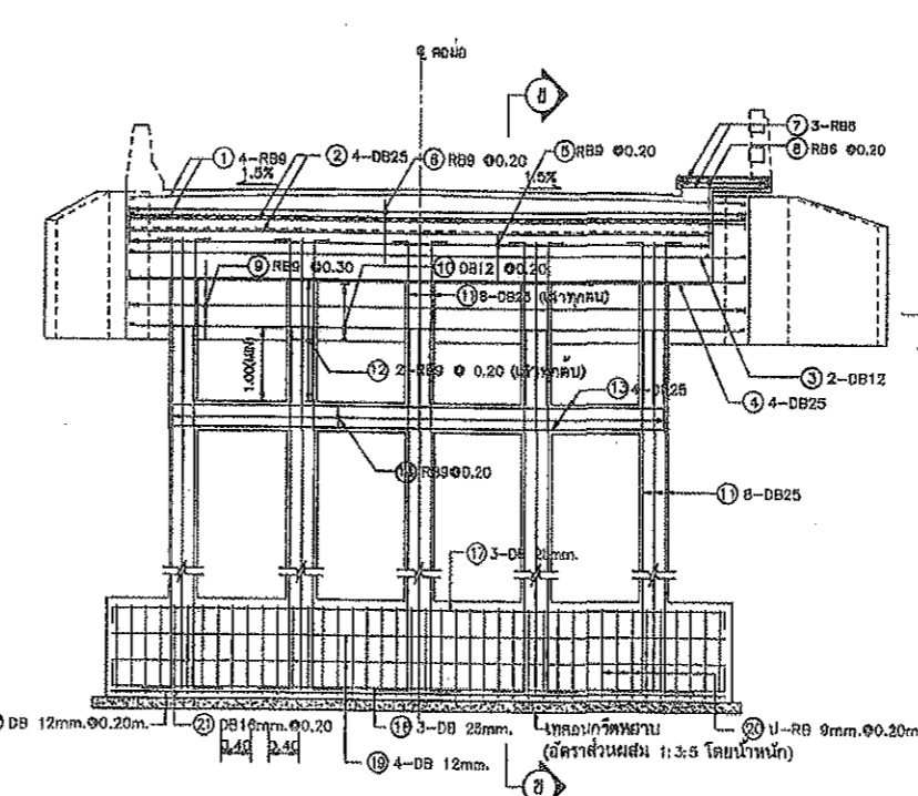
ครึ่งส่วนไม่มีทางเท้า ครึ่งส่วนมีทางเท้า แสดงภาพส่วนเหล็กค่อมอุ้งฐานแผ่ มาตราส่วนแบบที่ 1
