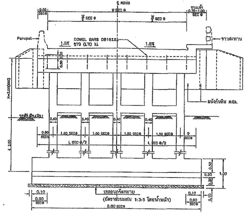
ครึ่งส่วน ไม่มีทางเท้า ครึ่งส่วนมีทางเท้า แสดงแปลนค่อมอุ้งฐานแผ่ มาตราส่วนแบบที่ 1
