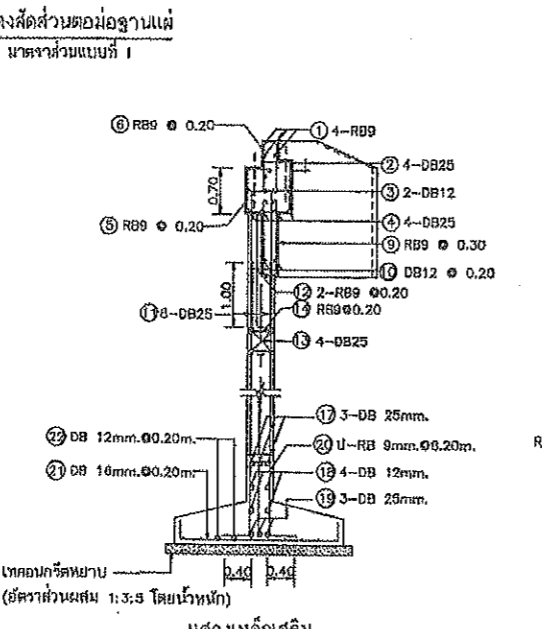
รูปตัด (B)-(B) มาตราส่วนแบบที่ 1
