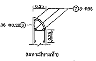
รายละเอียด (1) มาตราส่วนแบบที่ 2
