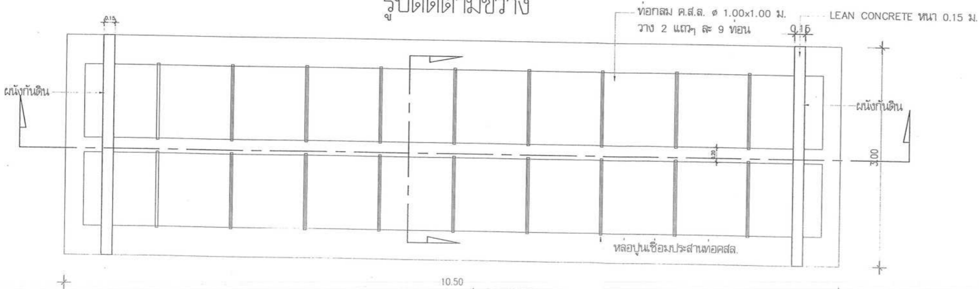
รูปแปลนวางท่อ ค.ส.ล.
