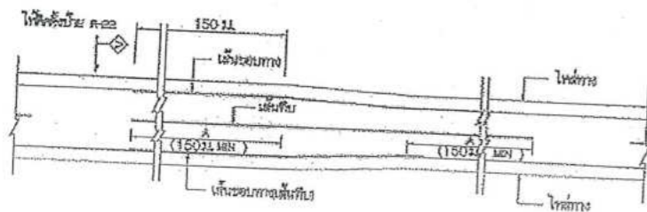
การขึ้นจราจร กรณีความกว้างของช่องจราจรลดลง
