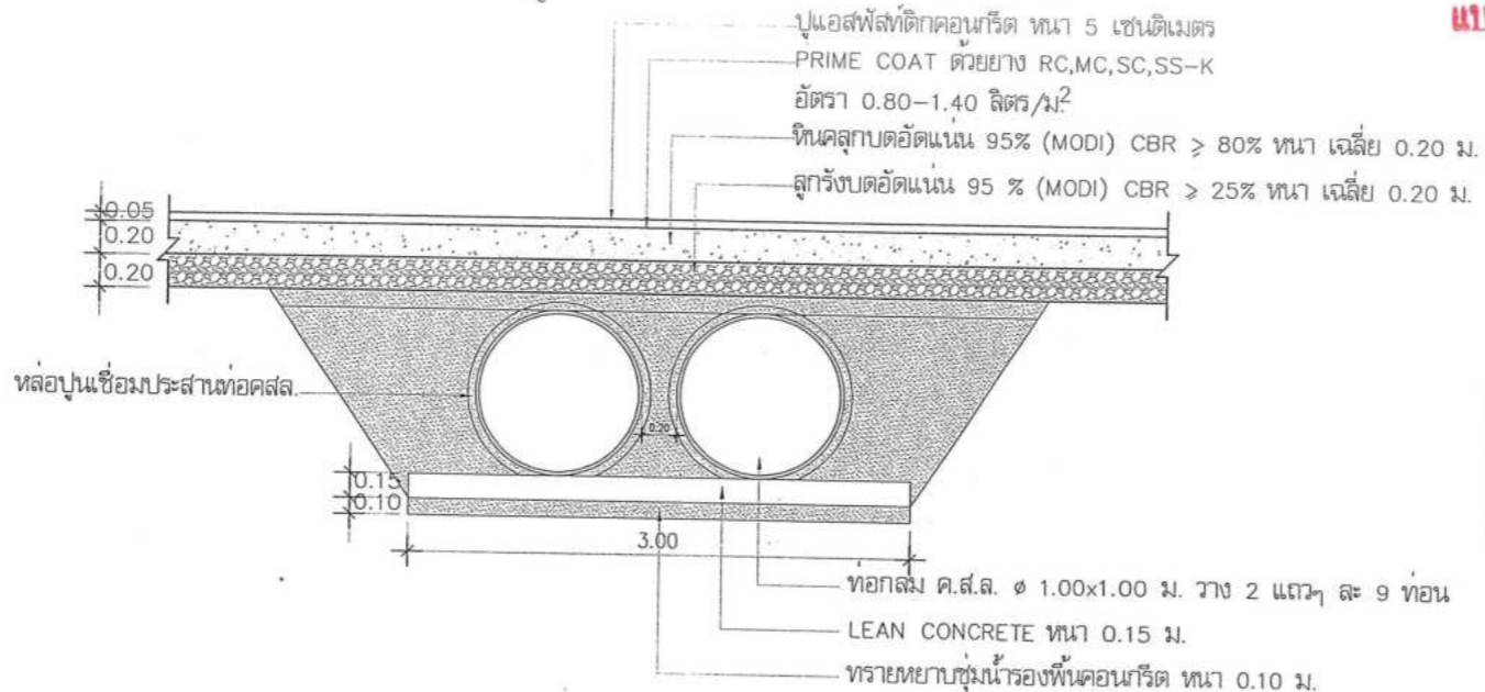
รูปตัดตามขวาง
