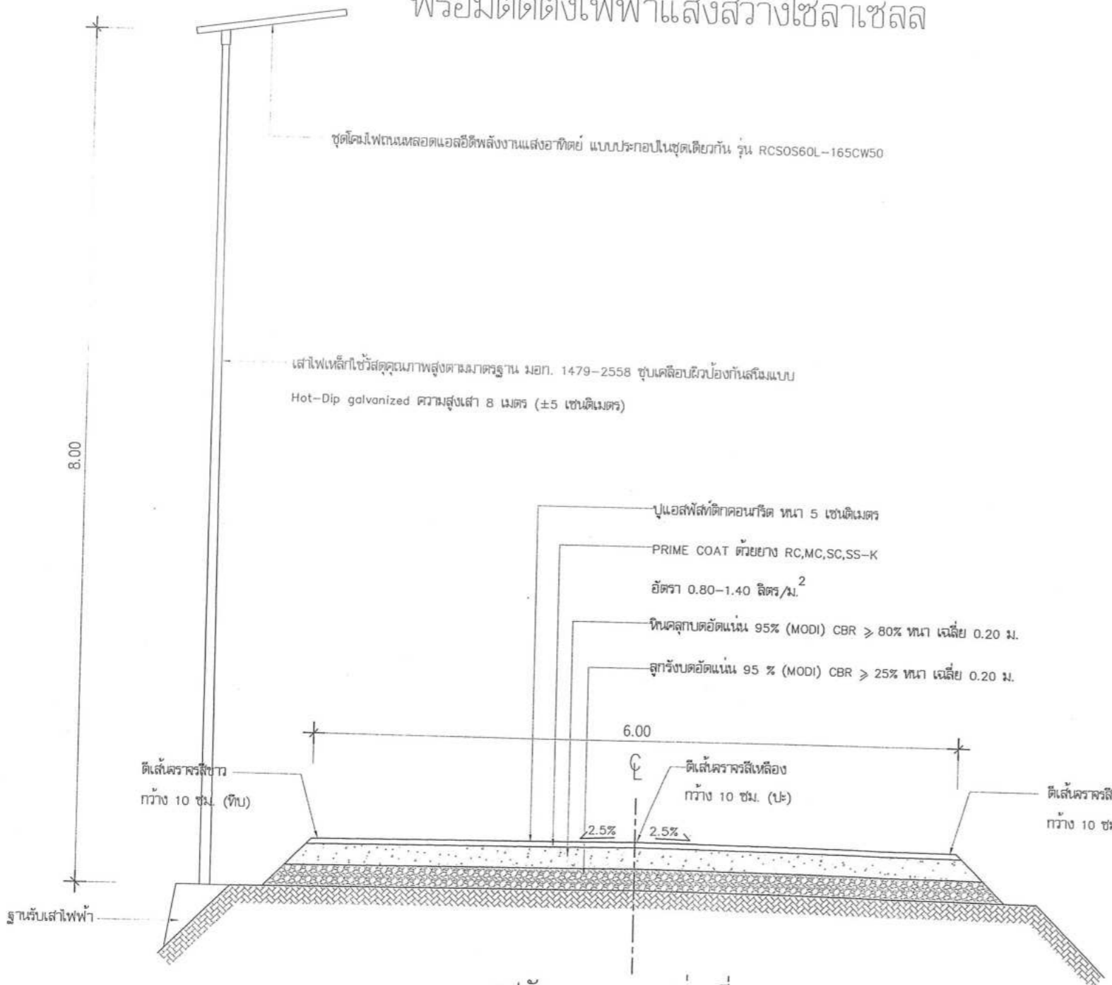
รูปตัดตามขวาง (ช่วงที่ 2) ก่อสร้างถนนลาดยางแบบแอสฟัลต์ติกคอนกรีต (Asphaltic Concrete)
