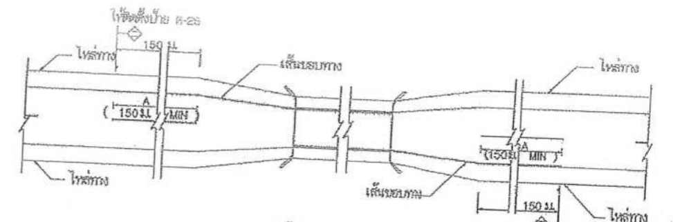
การขึ้นจราจรบริเวณสะพาน
