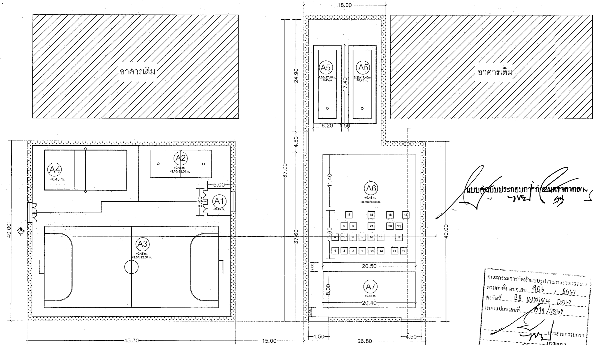
ผังบริเวณ มาตราส่วน 1 : 400
