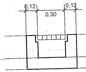
แบบขยาย : RC gutter
