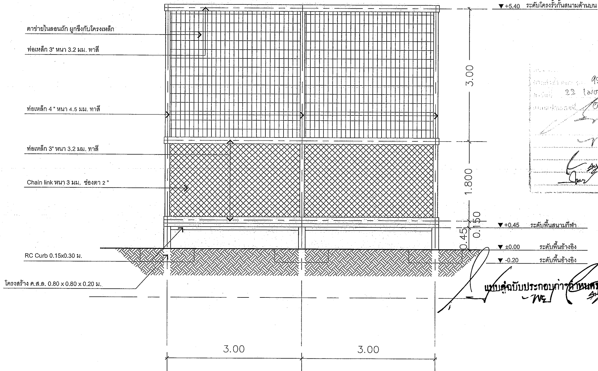
รั้ว 1 Unit แบบขยายรั้วกันสนาม มาตรฐาน 1 : 50
