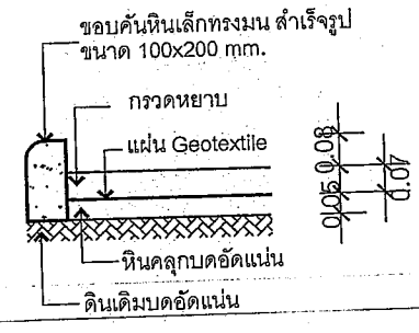
แบบขยาย - 01 : สนามเปิด
