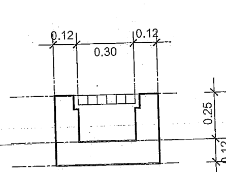
แบบขยาย : RC gutter
