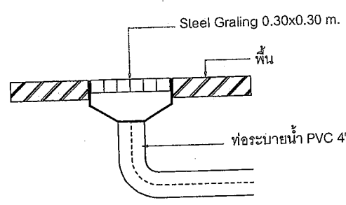
แบบขยาย Floor Drain
