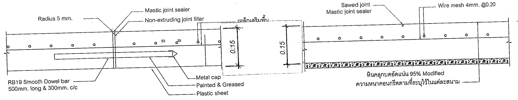
แบบขยายโครงสร้างพื้น : สำหรับพื้นที่ ค.ส.ล. ทั่วไป
