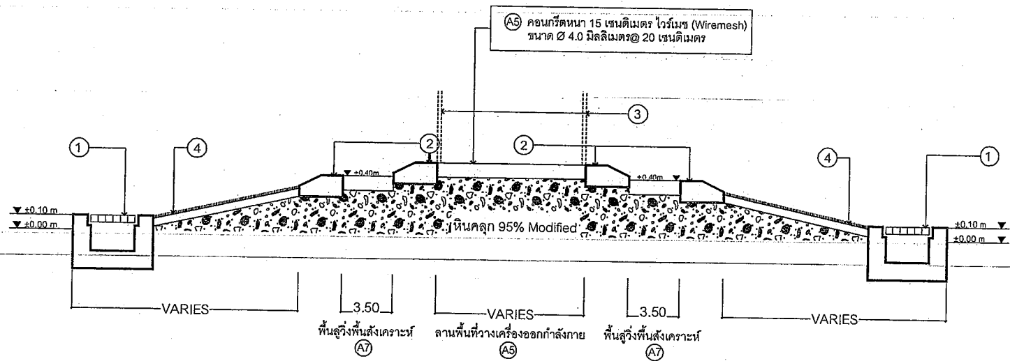
รูปตัด B
